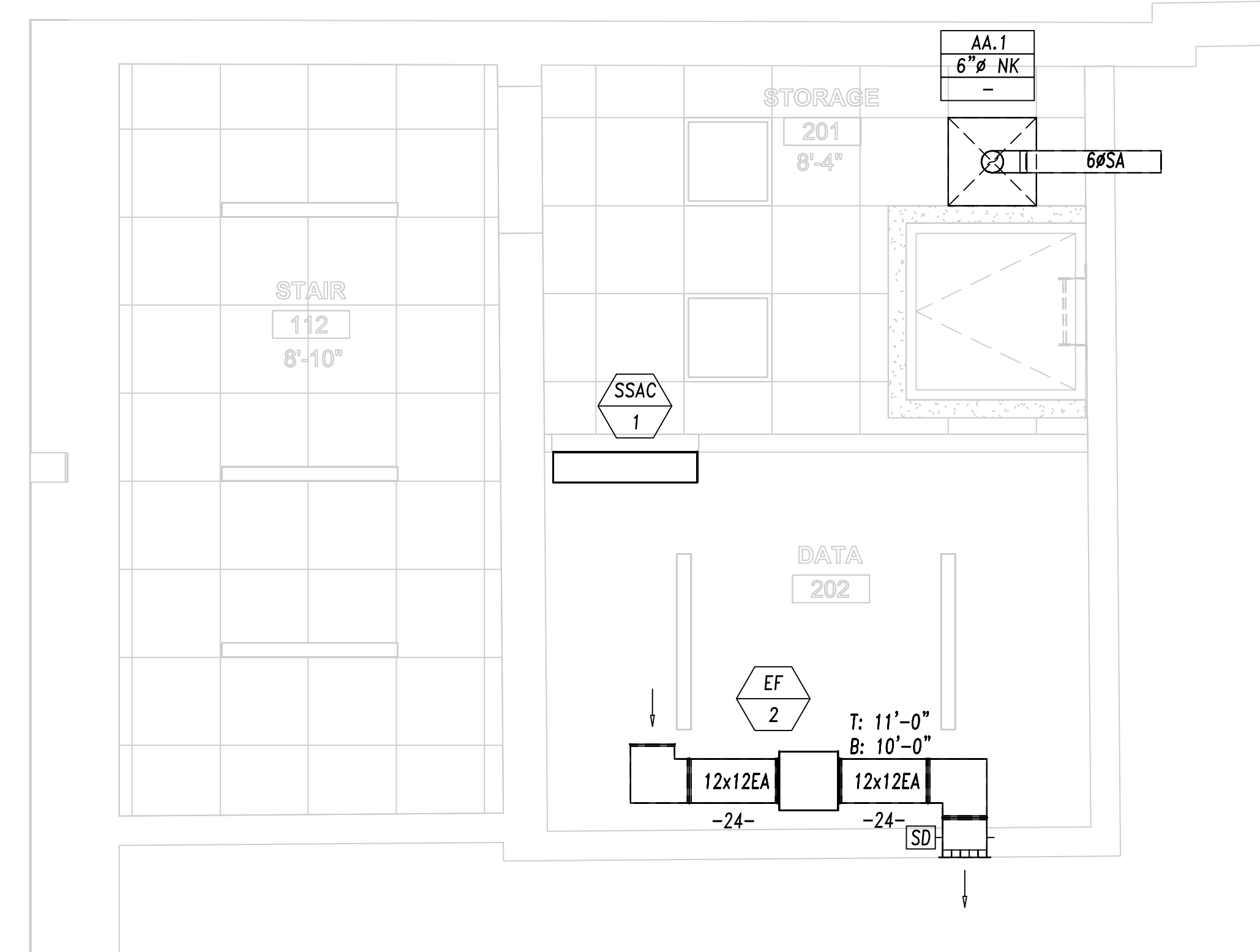
2 MEZZANINE HVAC PLAN SCALE: 1/4" = 1'-0"
